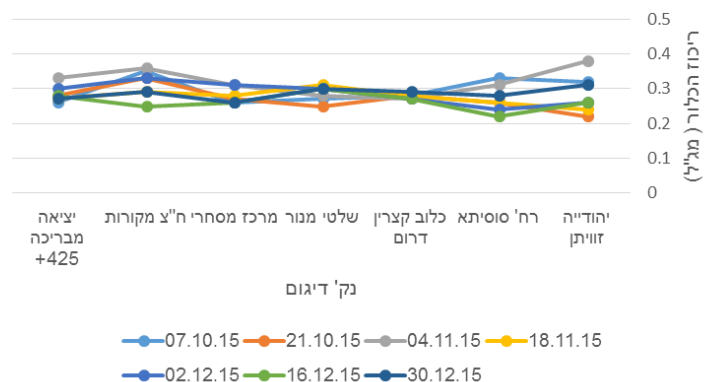
ריכוז הכלור בקצרין אוקטובר-דצמבר 2015
