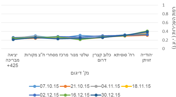
רמת העכירות בקצרין אוקטובר-דצמבר 2015
