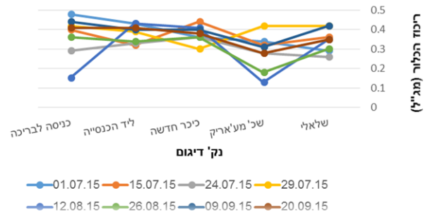
ריכוז הכלור בעין קיניא יולי - ספטמבר 2015
