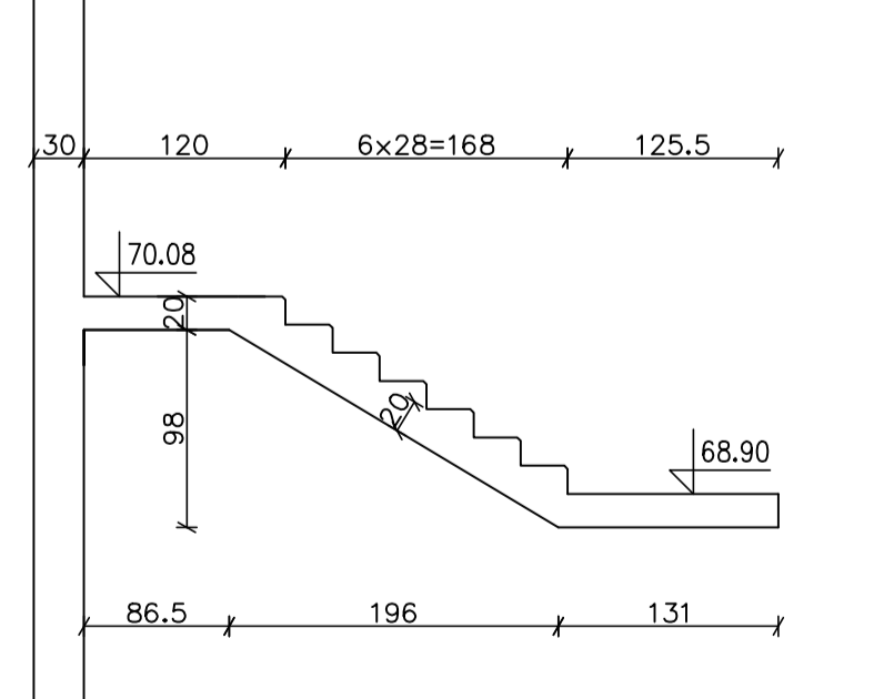
חתך G-G 1 : 50
